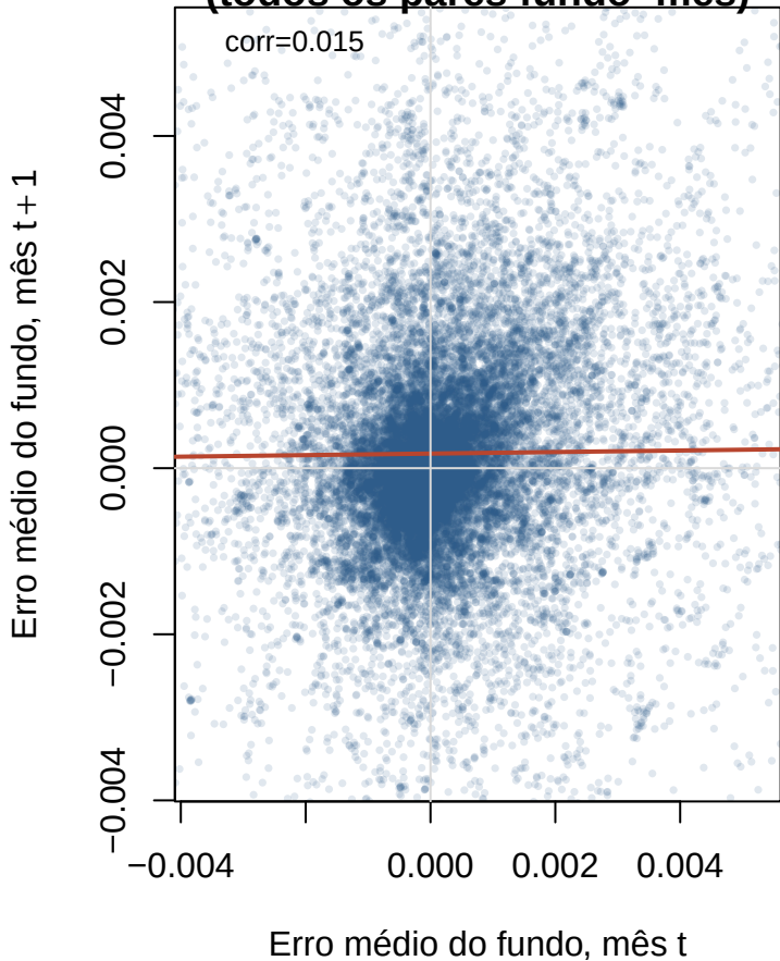
Erro consecutivo (todos os pares fundo-mês)
