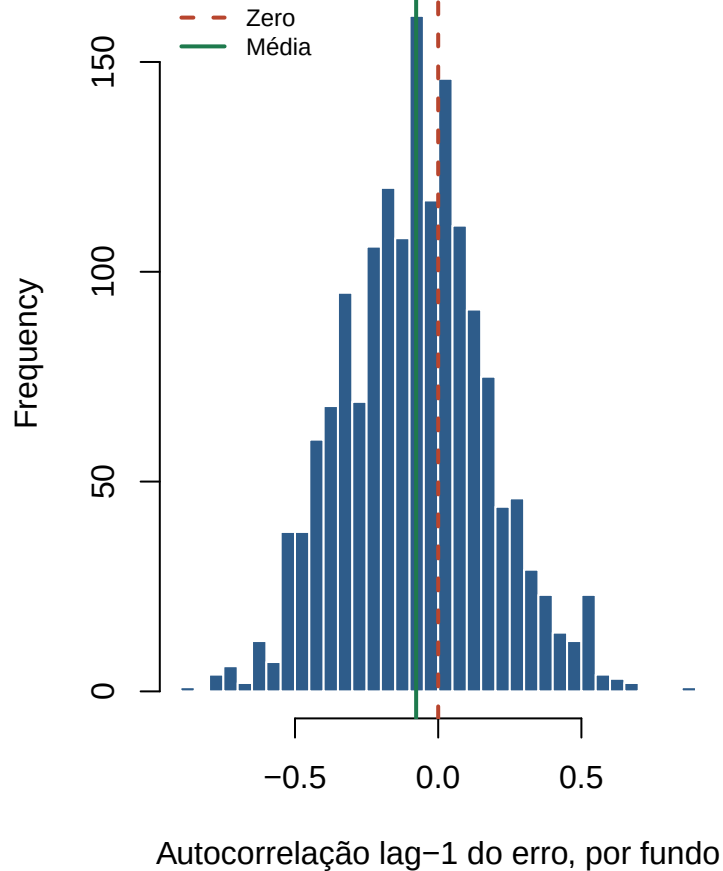
Distribuição entre fundos (=8 pares cada)
